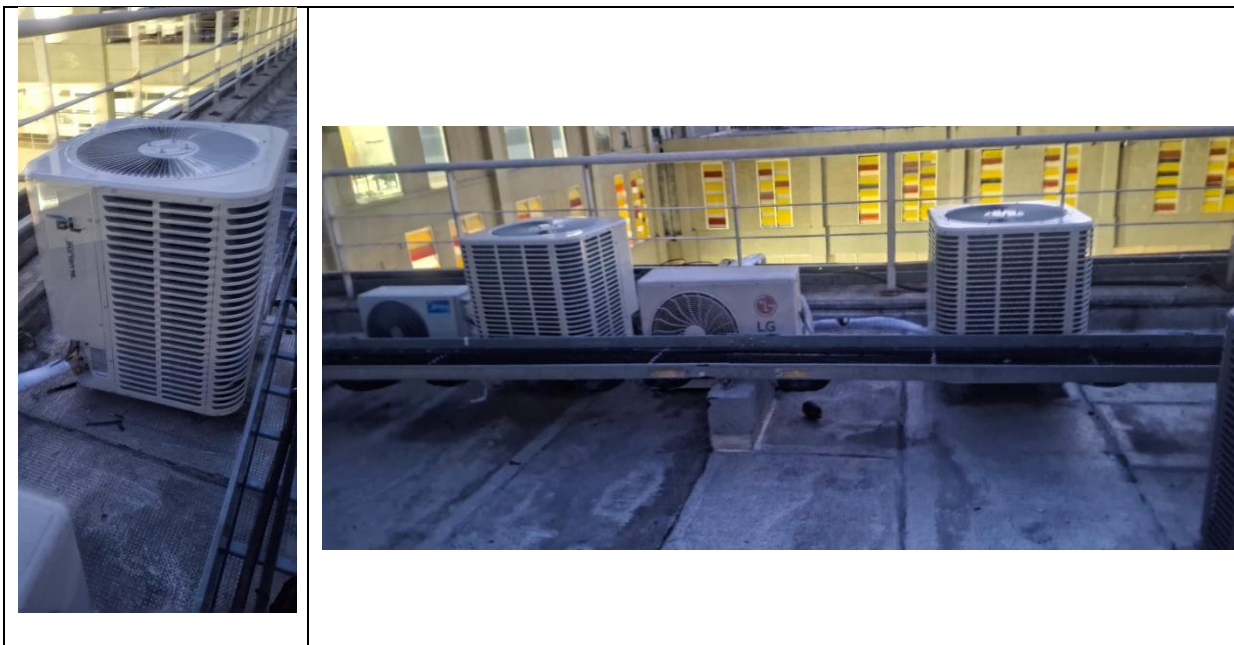
Condensadoras BlueLine Suministrados e Instalados
